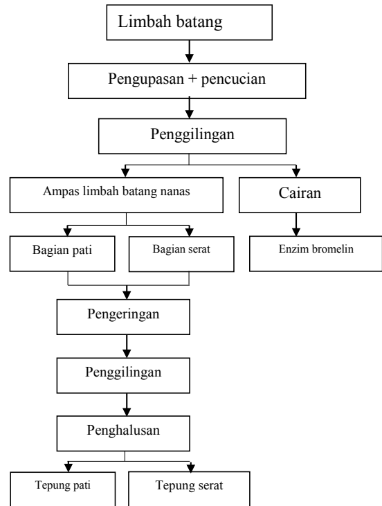
Gambar 1. Diagram alir proses pengolahan limbah batang nanas
