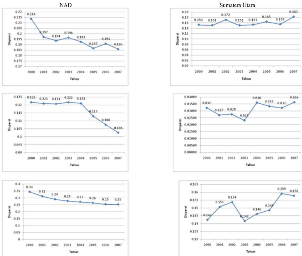
Gambar 4.1 Hasil Perhitungan Konvergensi di Pulau Sumatera
