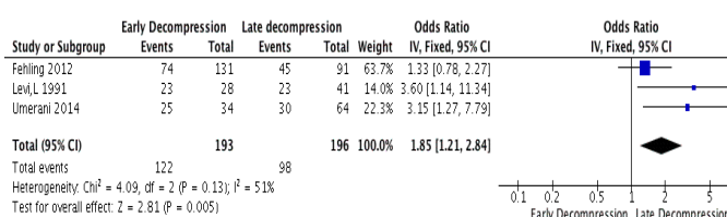
Gambar 2. Forest plot perbaikan status neurologis pada kelompok tindakan pembedahan dekompresi dini dan kelompok pembedahan dekompresi tertunda
